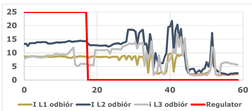
Przebiegi prądów po stronie odbiorców – wyłączenie regulatora w 17.sekundzie
