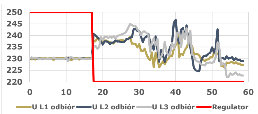
Przebiegi napięć po stronie odbiorców – wyłączenie regulatora w 17.sekundzie
